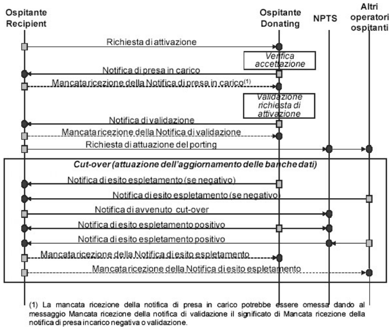
Figura 1- Sequenza dei messaggi nel caso di attivazione standard
